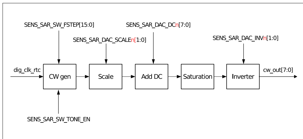
图 29-10. 余弦波形生成器的工作流程
