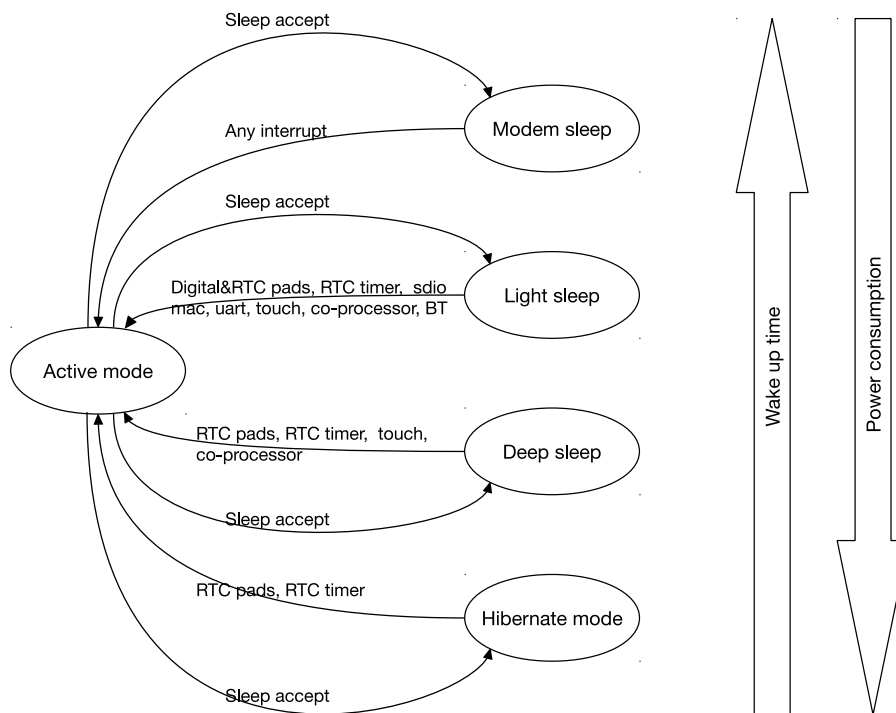
图 31-10. 功耗模式
