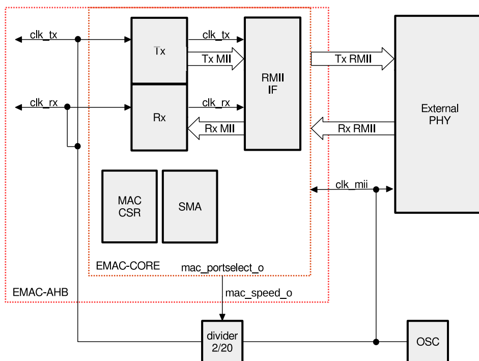
图 10-6. RMII 时钟
