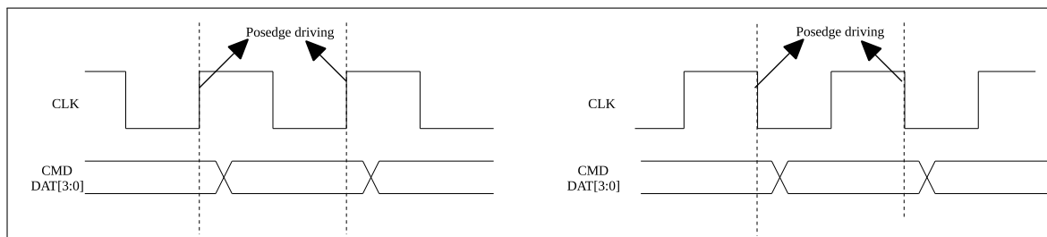
图 8-10. 输出时序图
