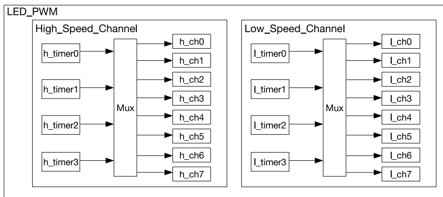
图 14-1. LED_PWM 架构
