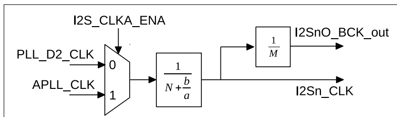
图 12-2. I2S 时钟
