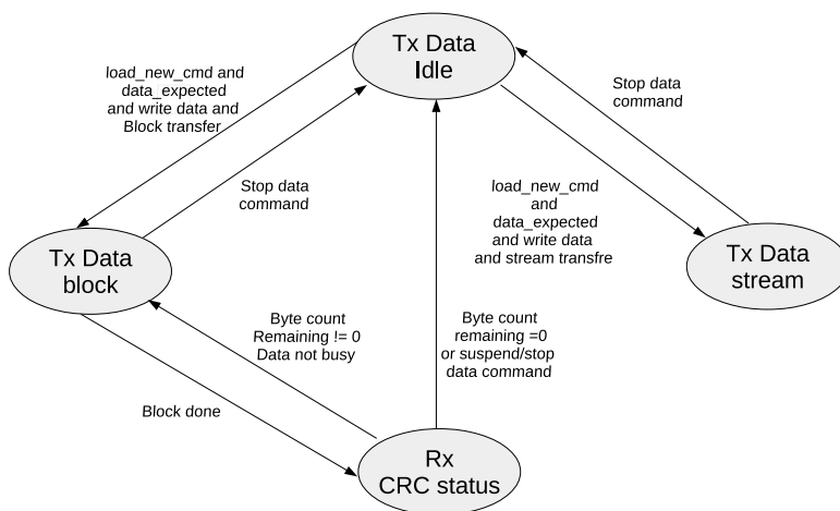
图 9-5. 数据传输状态机
