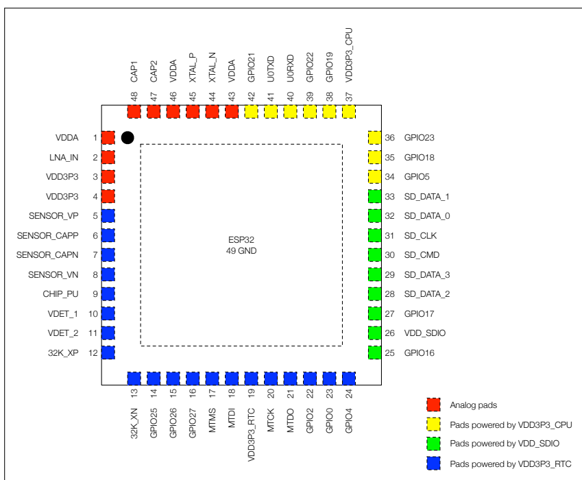
图 4-5. ESP32 GPIO 管脚供电电源 (QFN 6*6, 顶视图)
