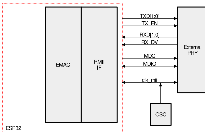
图 10-5. RMII 接口
