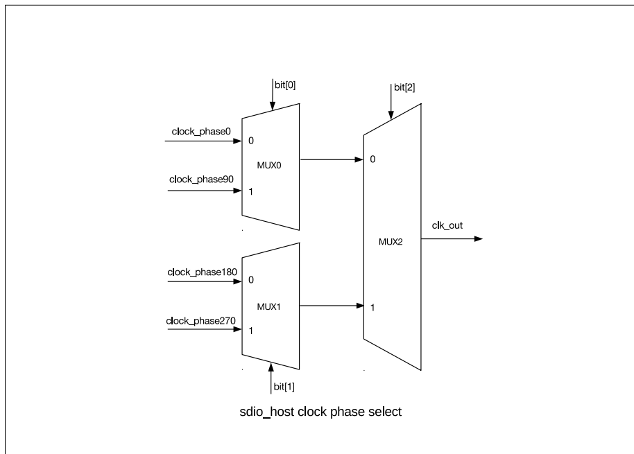
图 9-10. 时钟相位选择
