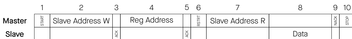
图 30-21. I2C 读操作
