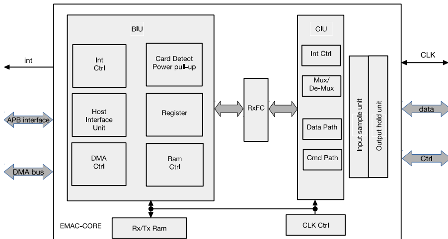
图 9-3. SD/MMC 基本架构
