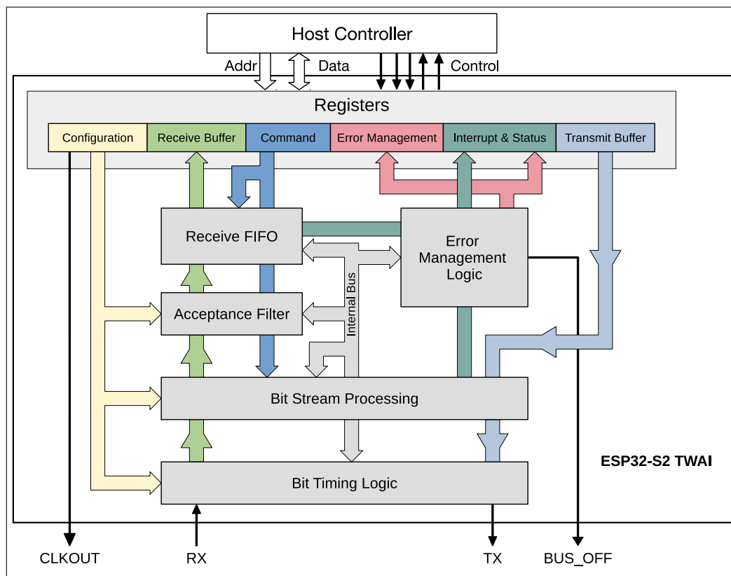
图 21-6. TWAI 概略图
