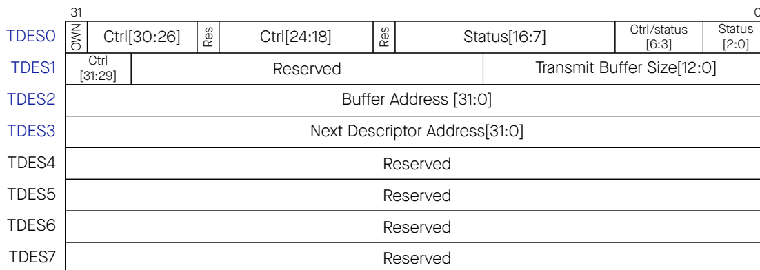
图 10-9. 发送描述符
