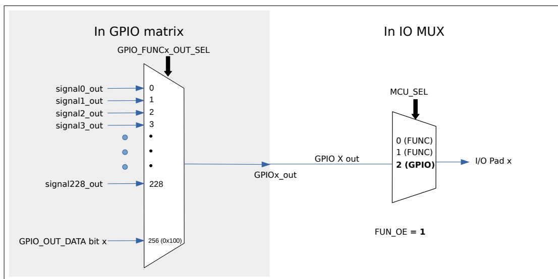
图 4-4. 通过 GPIO 交换矩阵输出信号
