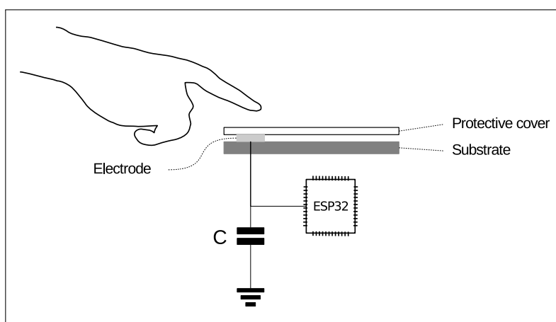
图 29-1. 触摸传感器
