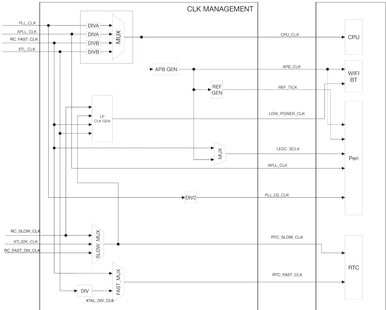
图 3-2. 系统时钟
