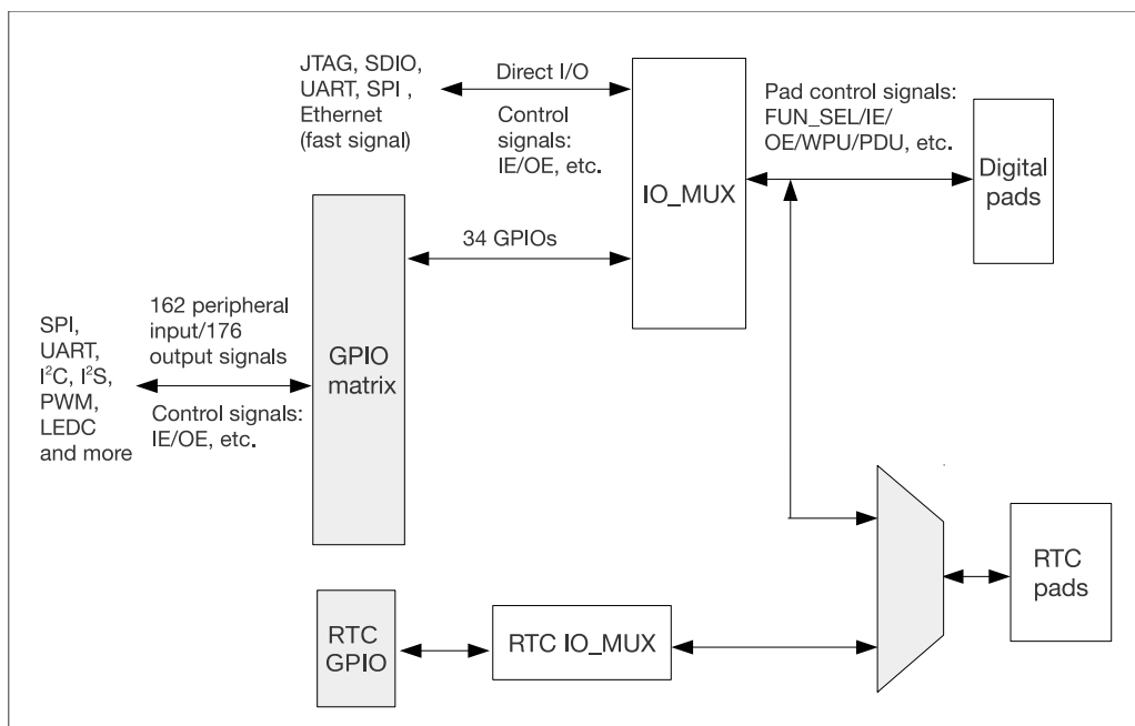
图 4-1. IO MUX、RTC IO MUX 和 GPIO 交换矩阵结构框图
