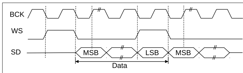
图 12-5. PCM 标准
