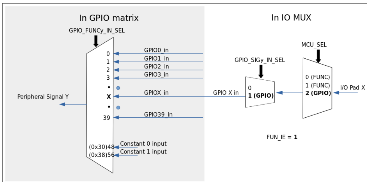
图 4-3. 通过 IO MUX、GPIO 交换矩阵的外设输入
