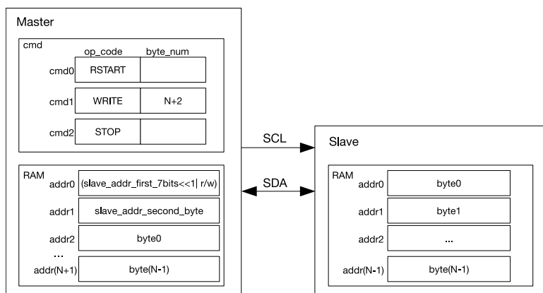
图 11-6. I2C Master 写 10-bit 地址 Slave
