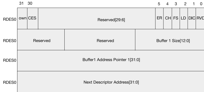
图 9-8. 链表结构
