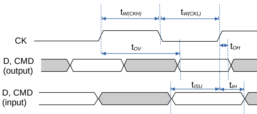
图 9-9. HS 模式下 SD/MMC 时序图
