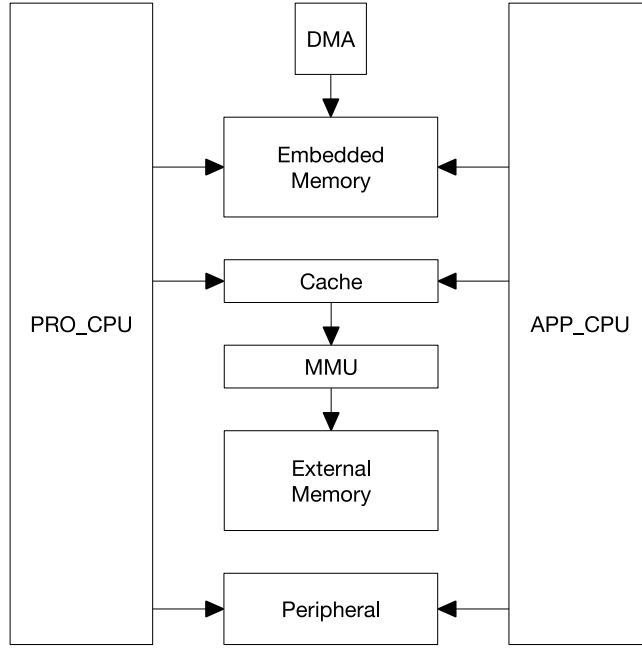
图 1-1. 系统结构
