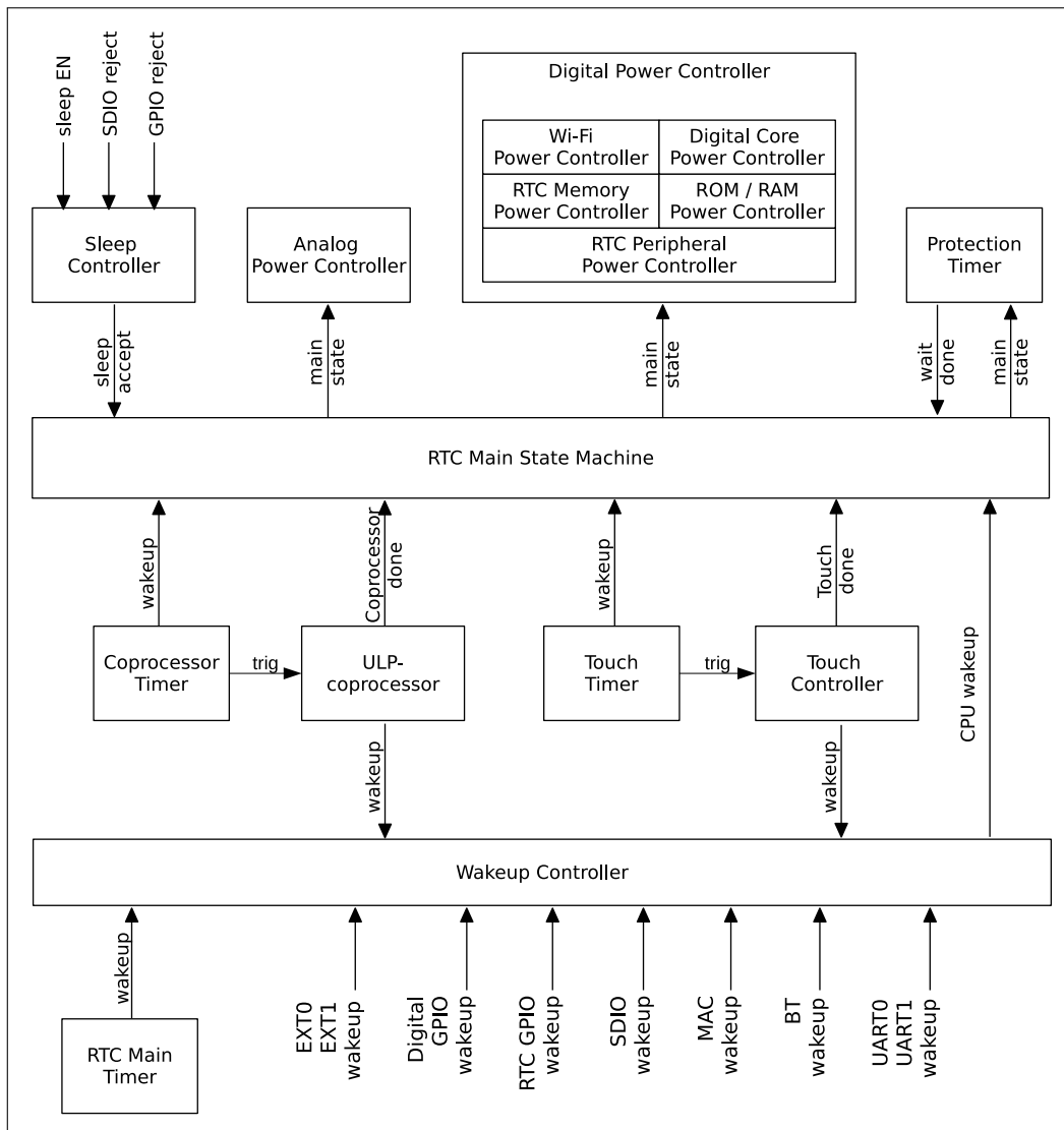
图 31-6. RTC 结构图
