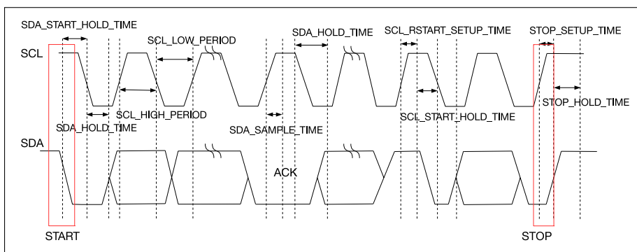
图 11-3. I2C 时序图
