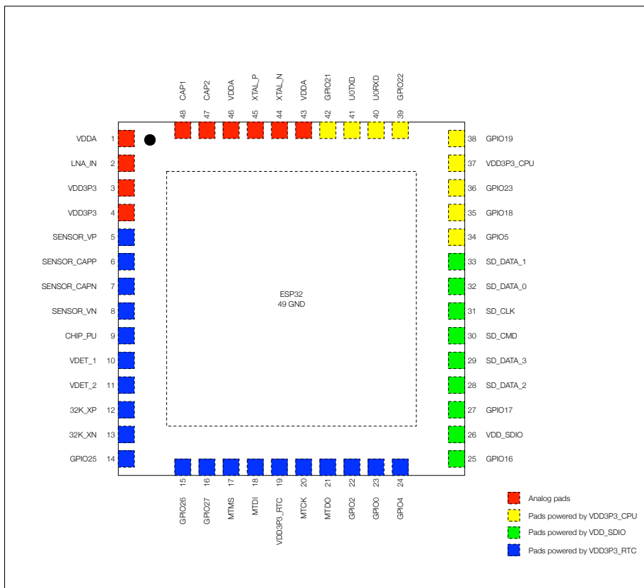
图 4-6. ESP32 GPIO 管脚供电电源 (QFN 5*5, 顶视图)
