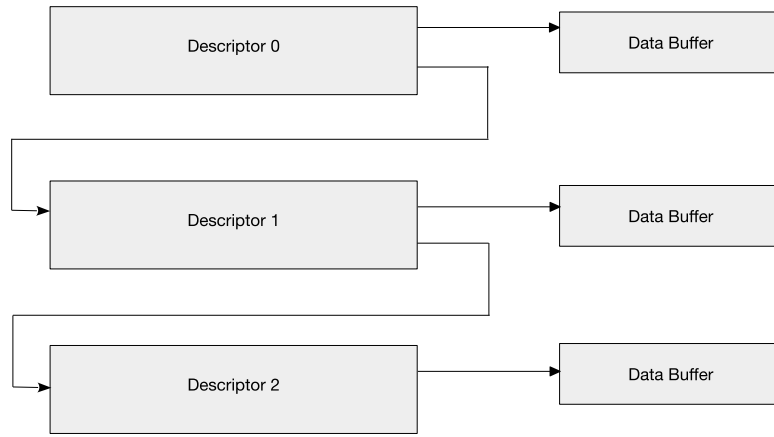
图 9-7. 链表环结构
