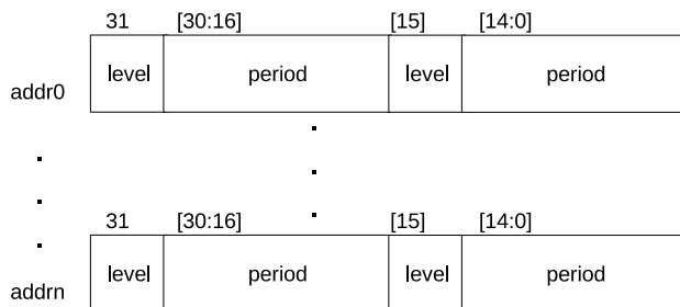
图 15-2. 数据结构
