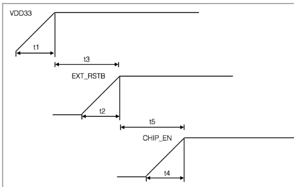
图 5-1. ESP8266EX 上电、复位时序图
