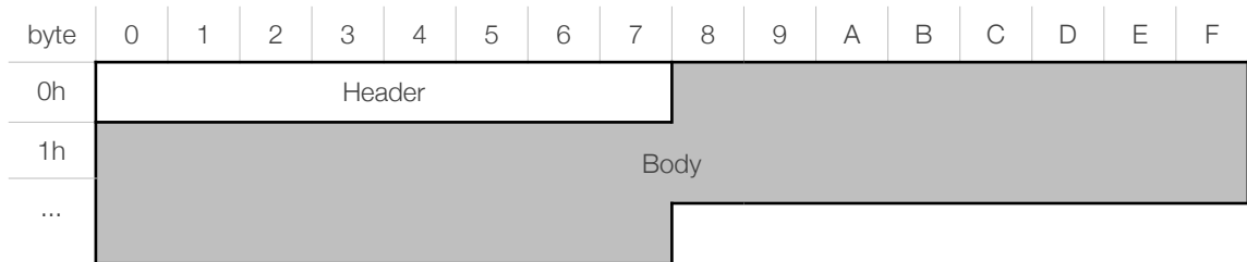
图 2-1. 数据包格式
