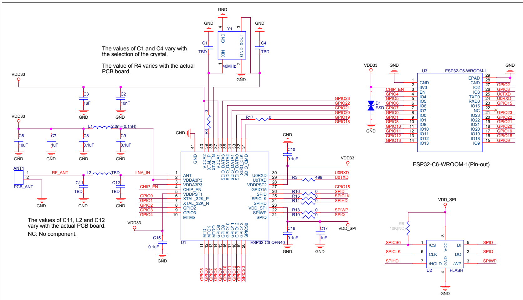
图 5: ESP32-C6-WROOM-1 原理图
