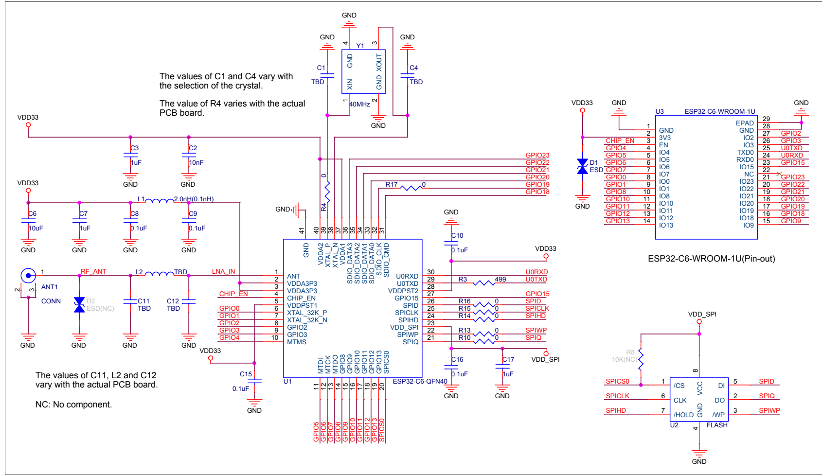
图 6: ESP32-C6-WROOM-1U 原理图
