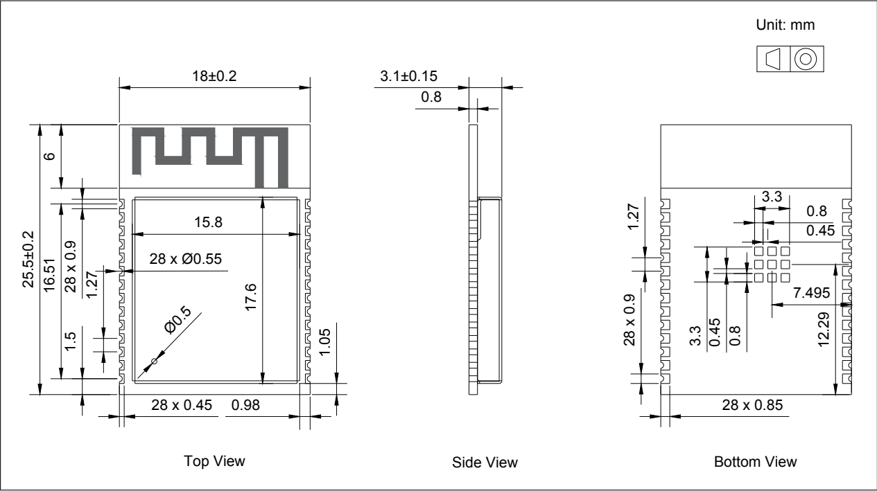
图 8: ESP32-C6-WROOM-1 模组尺寸
