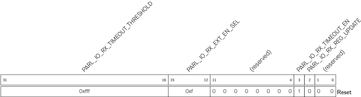
Register 38.2. PARL_IO_RX_CFG1_REG (0x0004)
