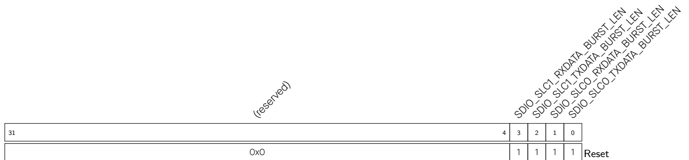
Register 34.29. SDIO_SLC_BURST_LEN_REG (0x017C)
