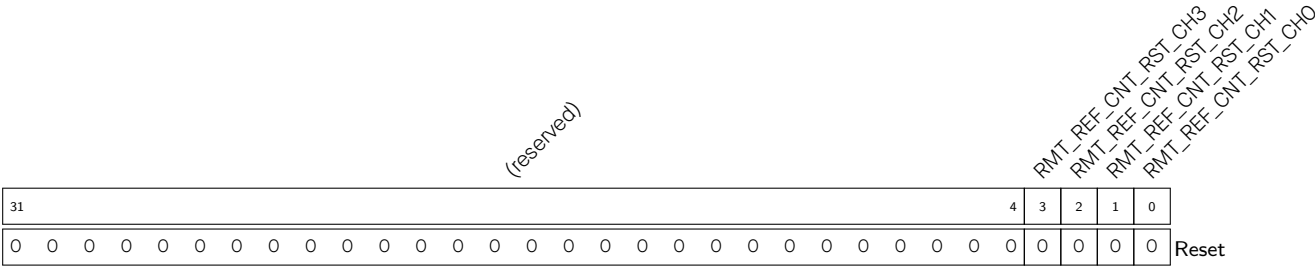
Register 37.6. RMT_REF_CNT_RST_REG (0x0070)
