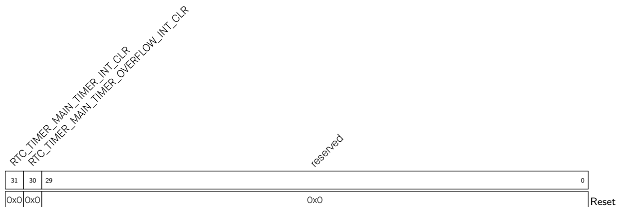
Register 12.75. RTC_TIMER_INT_CLR_REG (0x0034)
