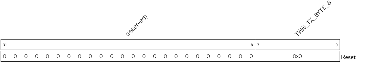
Register 33.13. TWAI_DATA_8_REG (0x0060)
