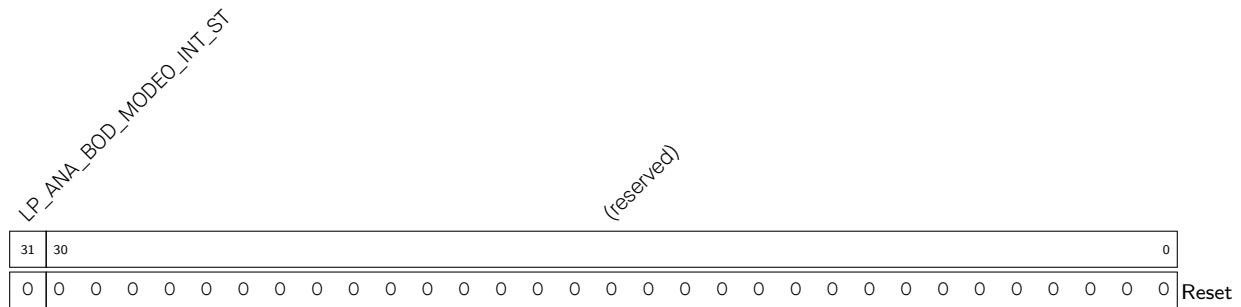
Register 12.84. LP_ANA_INT_ST_REG (0x0014)
