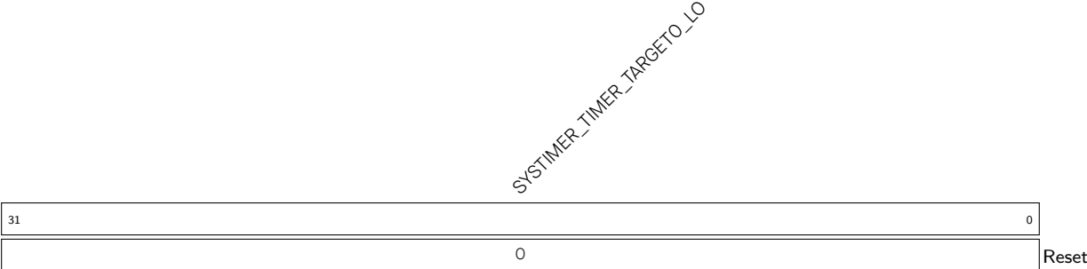
Register 13.15. SYSTIMER_TARGETO_LO_REG (0x0020)
