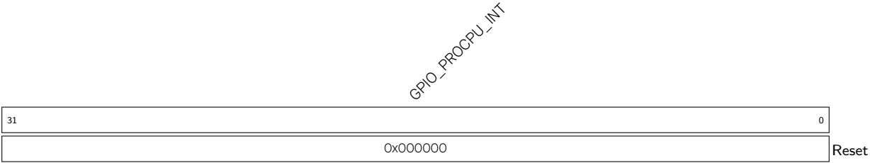
Register 7.12. GPIO_PCPU_INT_REG (0x005C)
