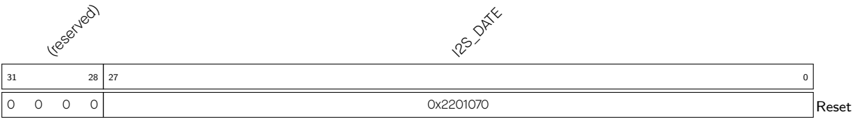
Register 30.20. I2S_DATE_REG (0x0080)
