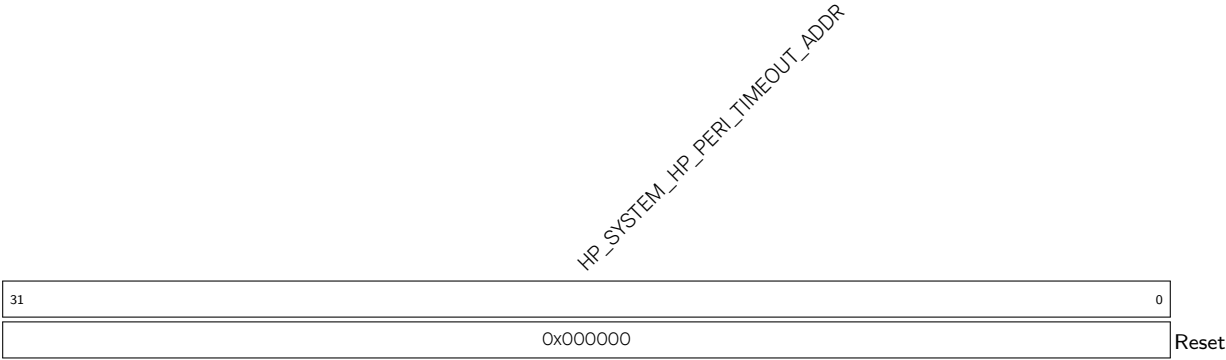
Register 17.8. HP_SYSTEM_HP_PERI_TIMEOUT_ADDR_REG (0x001C)
