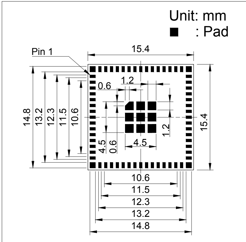
图 11: ESP32-S2-MINI-1U PCB 封装图形
