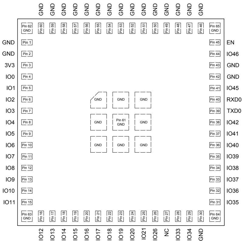
图 4: ESP32-S2-MINI-1U 管脚布局 (顶视图)
