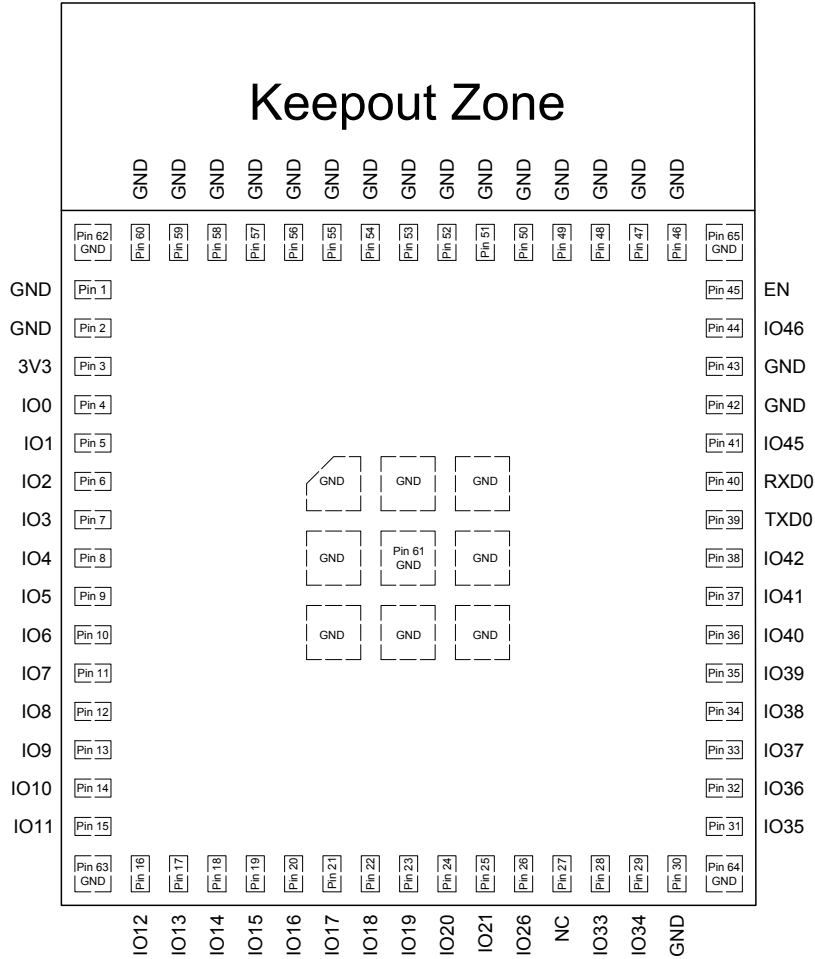
图 3: ESP32-S2-MINI-1 管脚布局 (顶视图)
