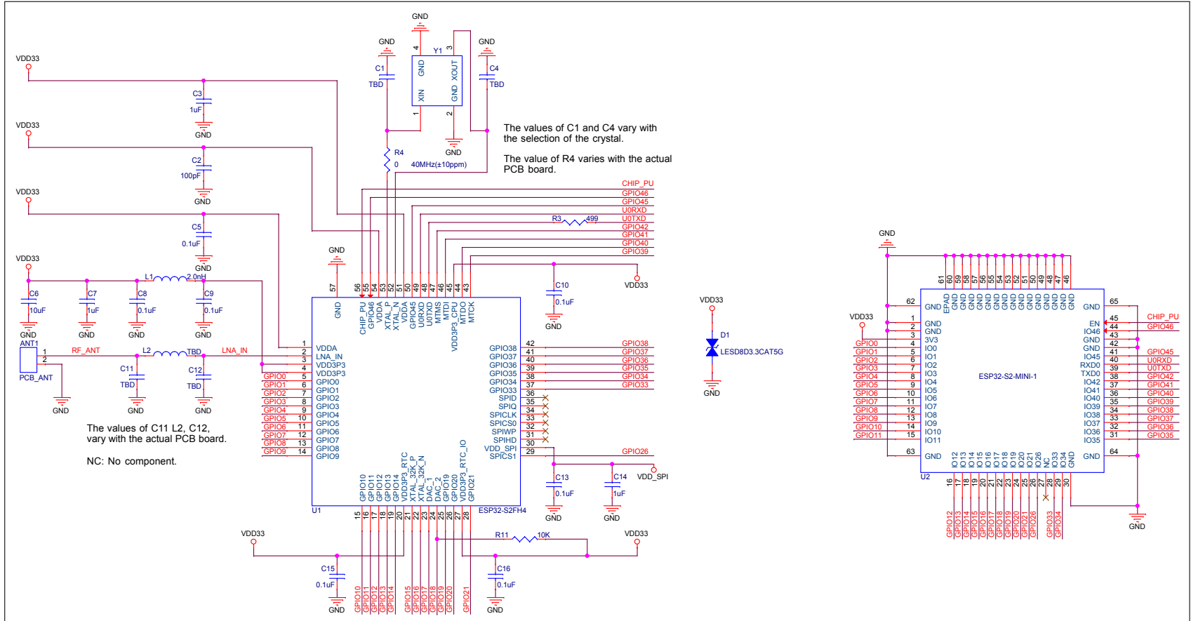
图 5: ESP32-S2-MINI-1 模组原理图
