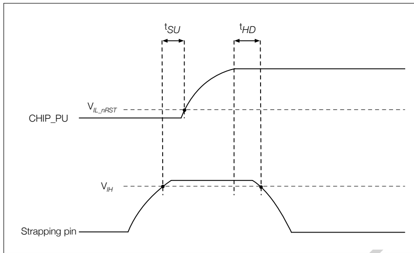
图 3: Strapping 管脚的建立时间和保持时间
