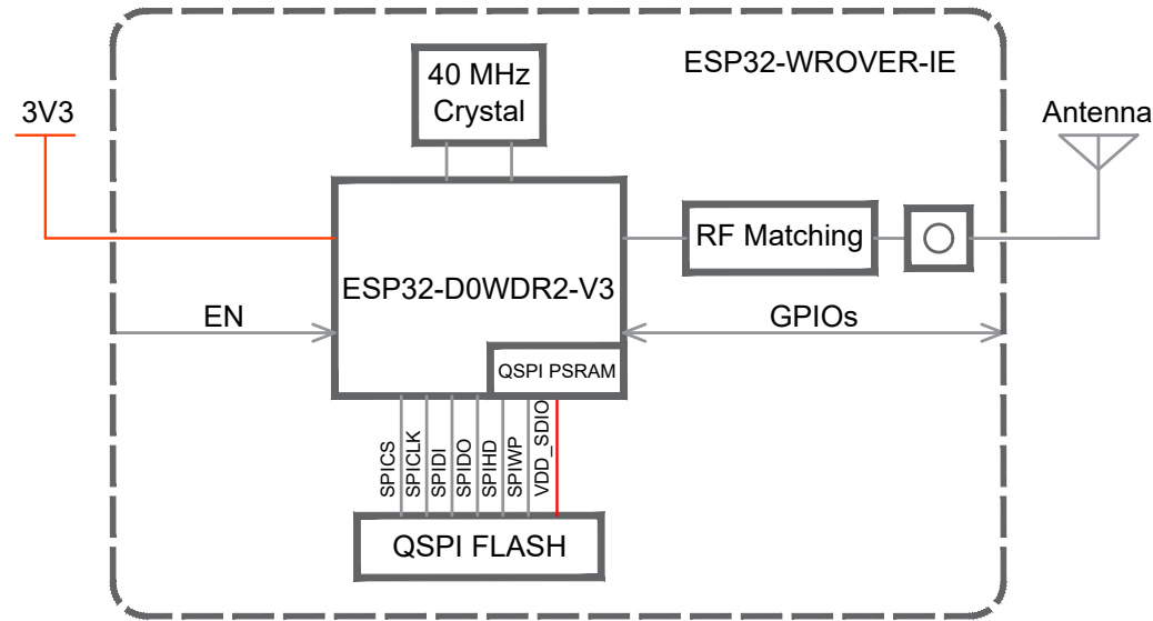
图 4: ESP32-WROVER-IE 模组功能框图（内置 ESP32-D0WDR2-V3 芯片）
