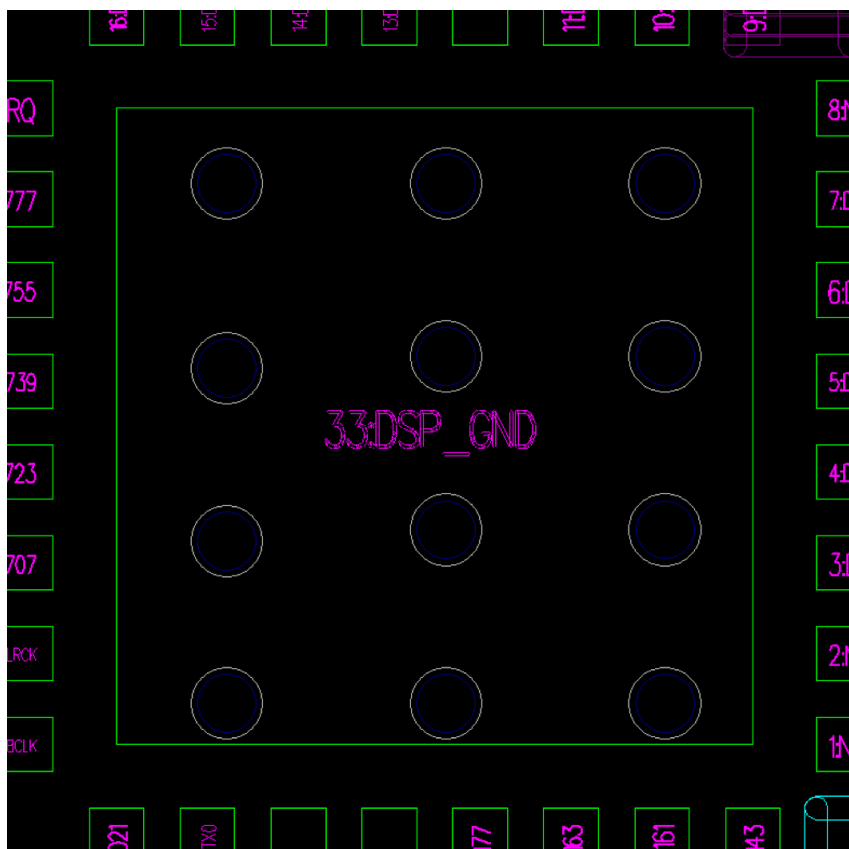
图 2-13. 地走线示例
