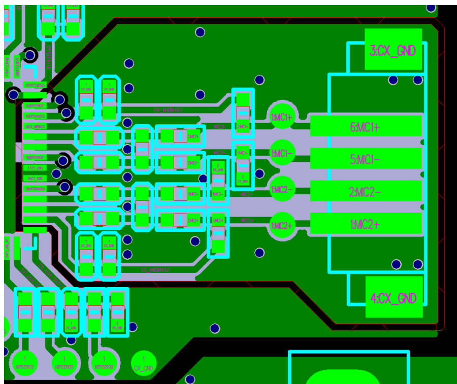
图 2-12. 地走线示例
