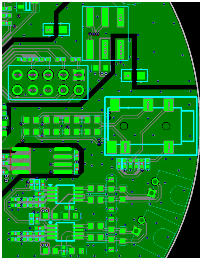
图 2-11. 地走线示例
