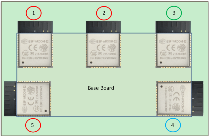
图 2-3. 模组位置摆放示例
