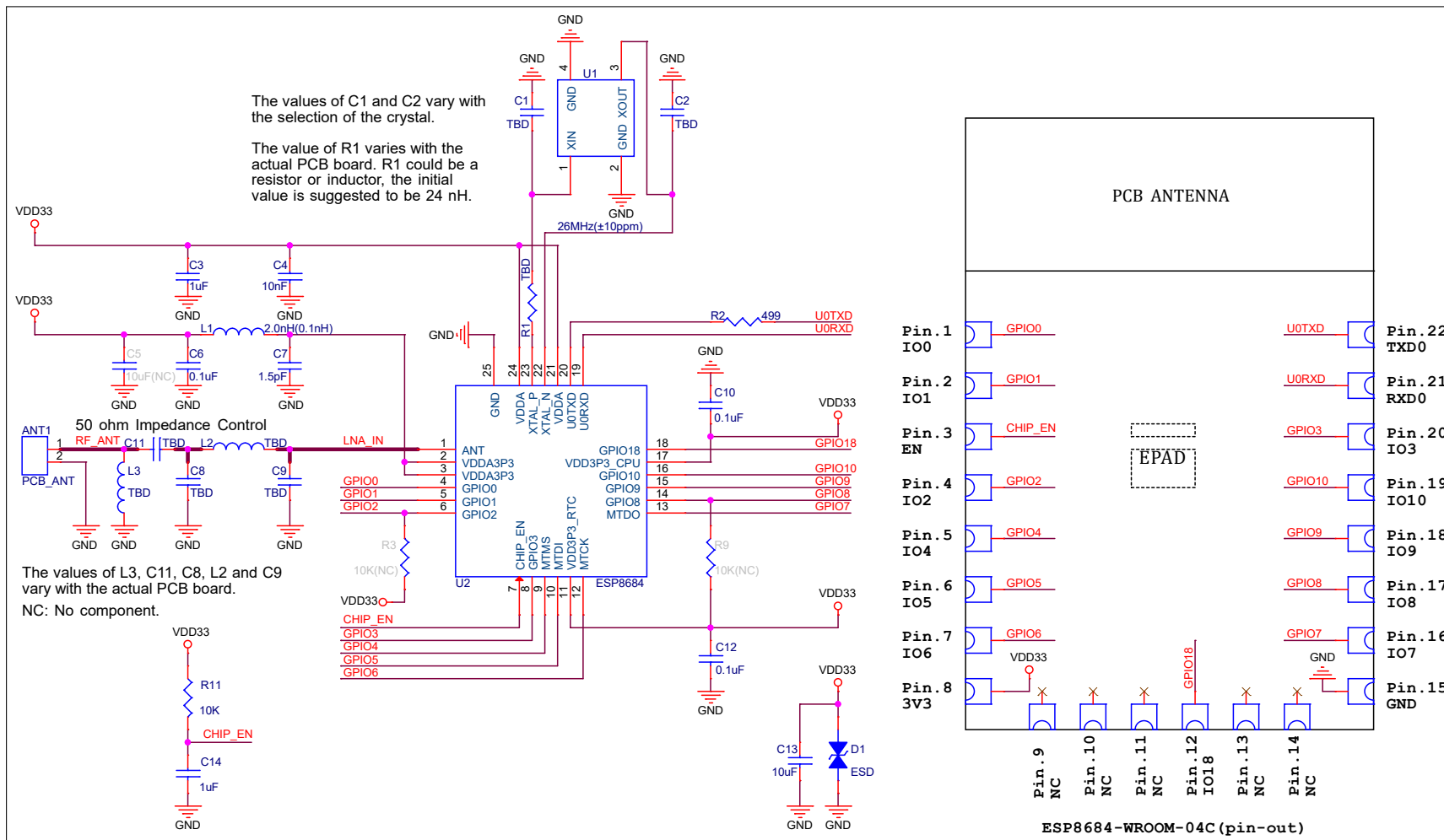
图 4: ESP8684-WROOM-04C 原理图
