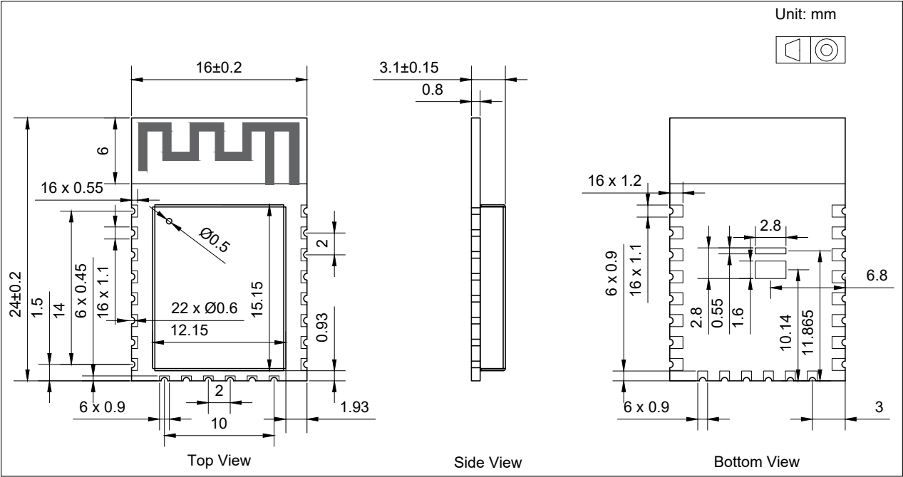
图 6: 模组尺寸
