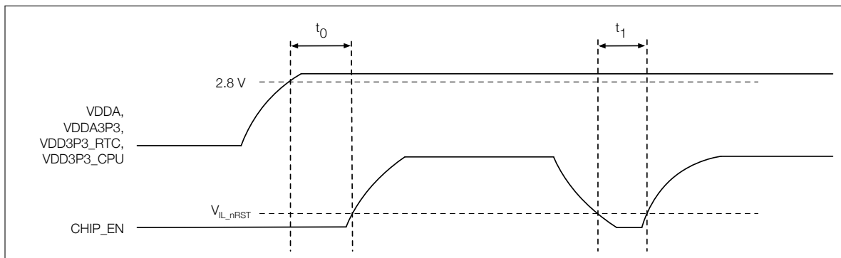
图 5: ESP8684 系列芯片上电、复位时序图
